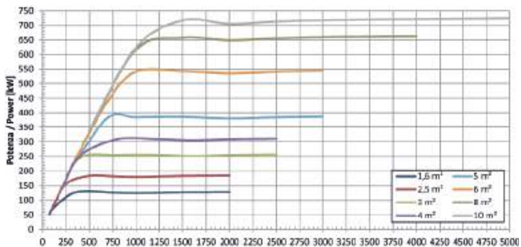
Portata al serpentino [L/h]
