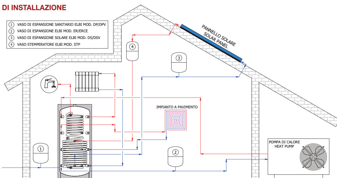
Schema illustrativo; per la realizzazione degli impianti fare sempre riferimento a tecnico abilitato.
