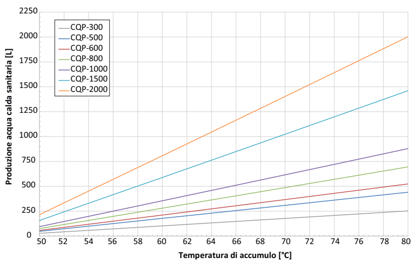
Produzione teorica acqua sanitaria (ingresso 10 °C, uscita 45 °C)
