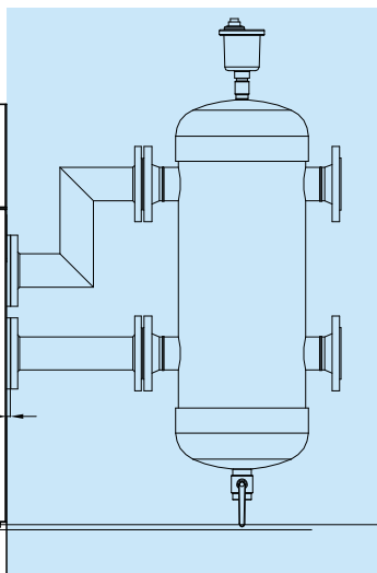
Centrale termica con separatore idraulico
