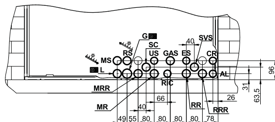
Installazione posteriore (vista frontale)
