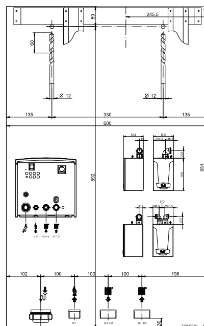
Dima di montaggio
