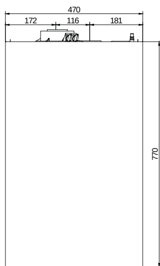
vista frontale
