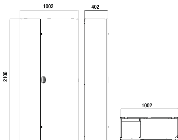
Installazione con armadio tecnico di contenimento (per versione CSI IN E - CSI IN Alya/Auriga E 200)
