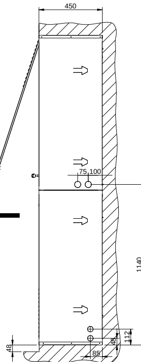
LATO DESTRO (vista da ext. cassa)
