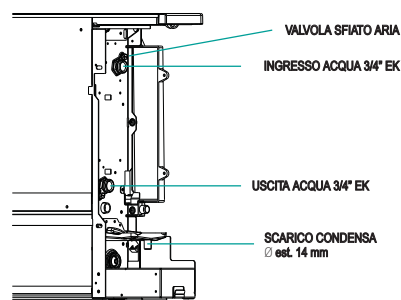
Attacchi idraulici
