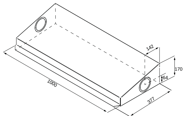
Kit copertura armadio tecnico
