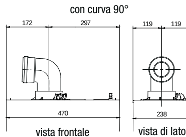
Luna IN Plus (installazione pensile) Luna Air (installazione pensile)
