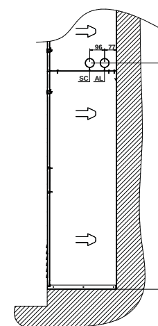
Connessioni laterali lato destro (vista da esterno cassa)
