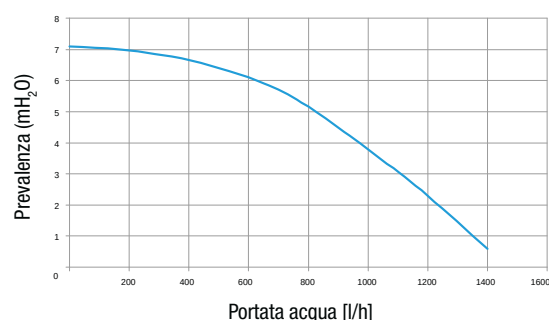
Pompa kit zona miscelata
