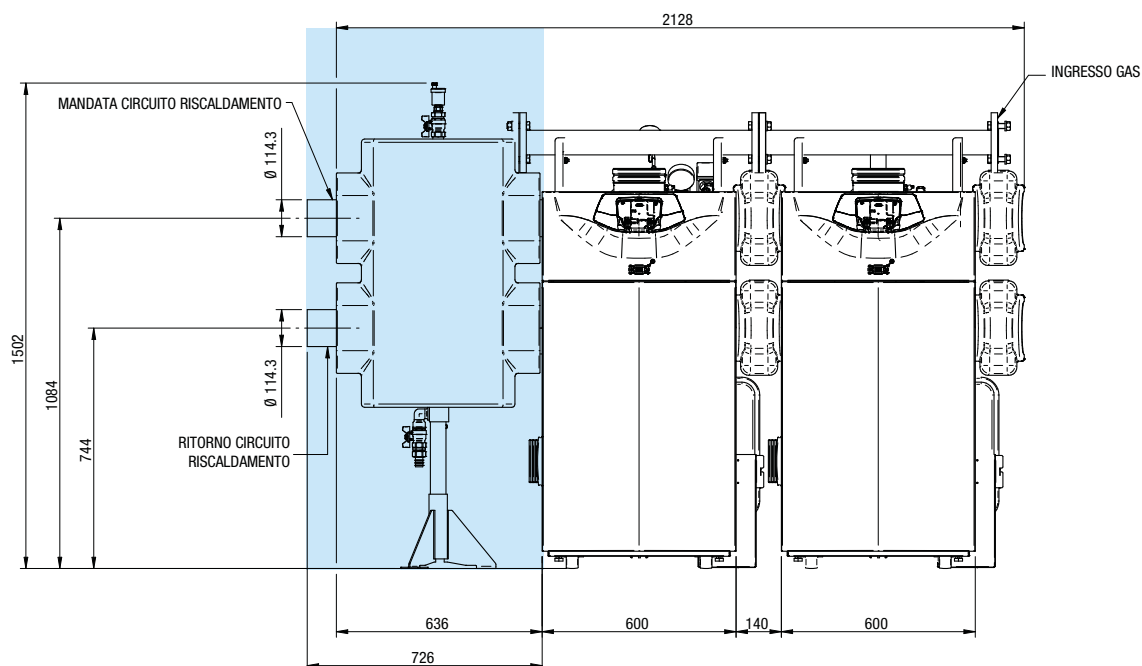
Centrale termica con separatore idraulico
