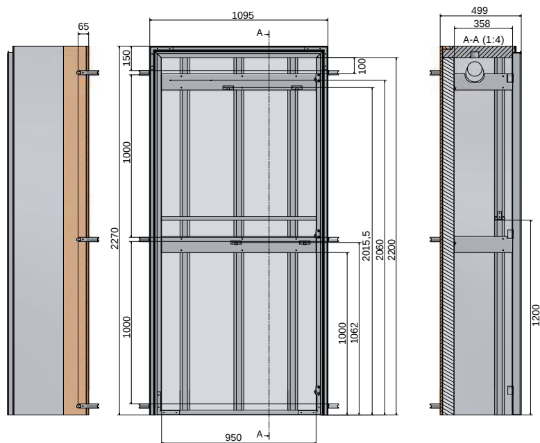
Cassa di contenimento isolata CSI IN (per versione CSI IN E / CSI IN E 200)
